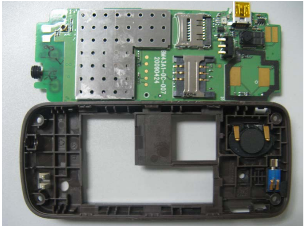
(10) EUT Photo
