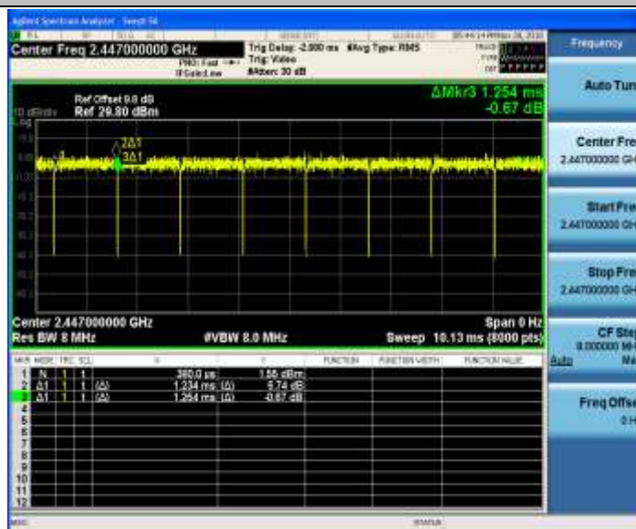
11N40MIMO_Ant2_2447
