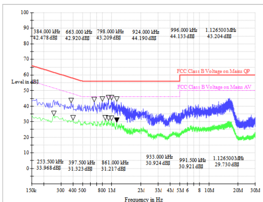
(Plot B: N Phase)
