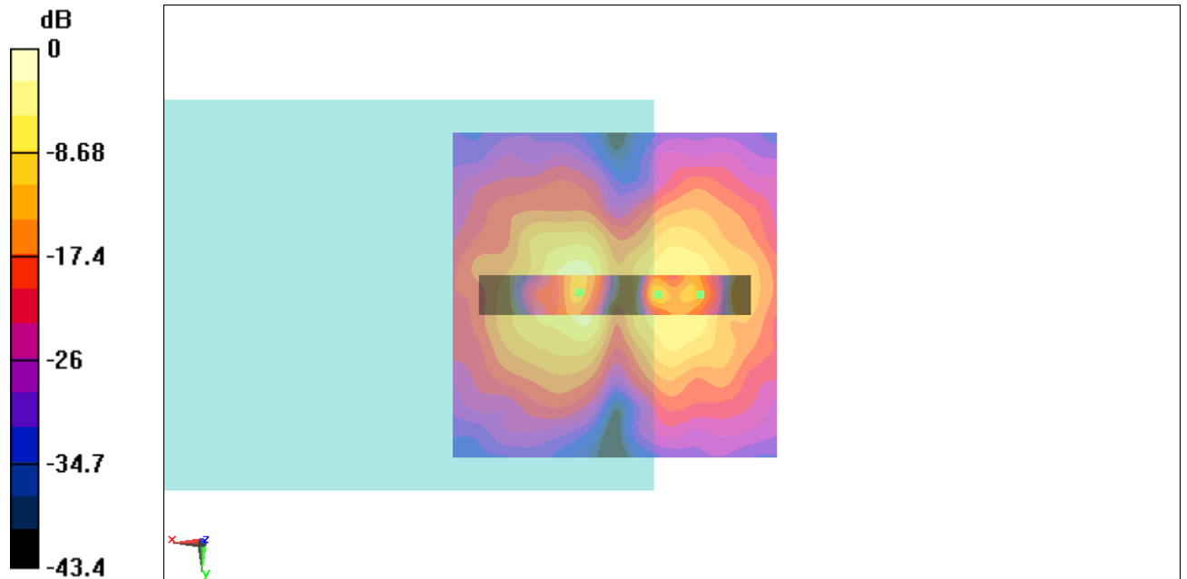
Fig B.4 T-Coil CDMA 835_Channel 384
