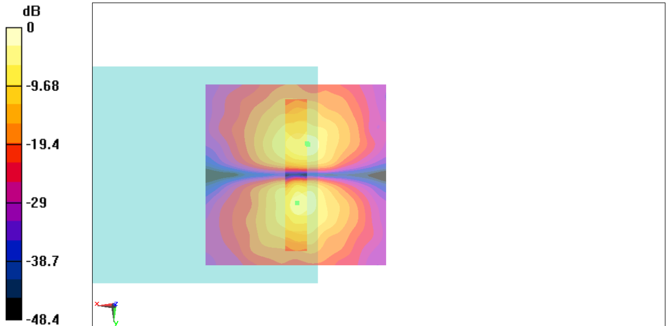
Fig B.5 T-Coil CDMA 835_Channel 384
