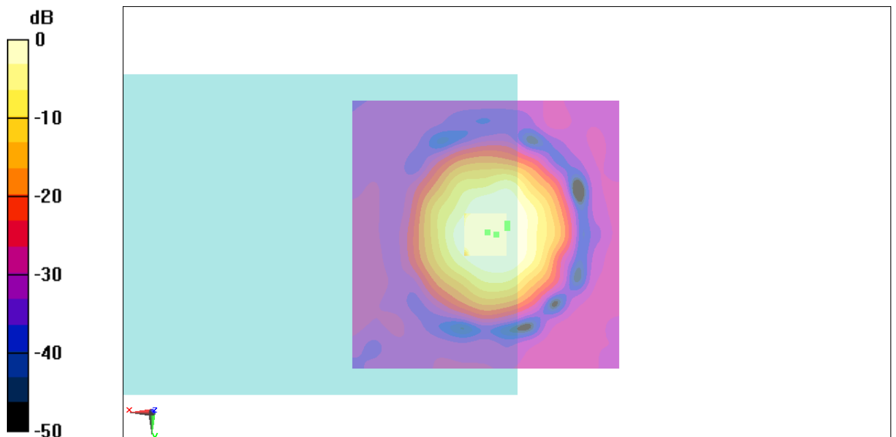
Fig B.6 T-Coil CDMA 835_Channel 384
