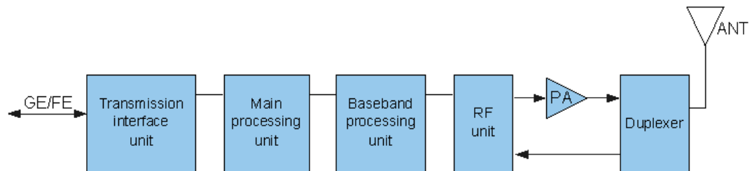
01 BTS3902E Structure
