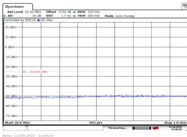
CA_7C 20MHz+10MHz CH- Middle 30MHz~1GHz
