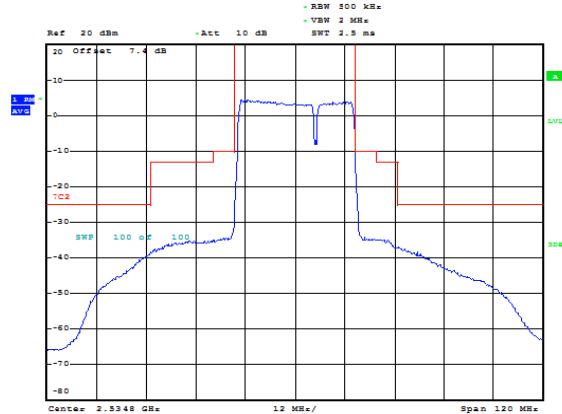
CA_7C 20MHz+10MHz QPSK RB=100#0+50#0 CH- Middle
