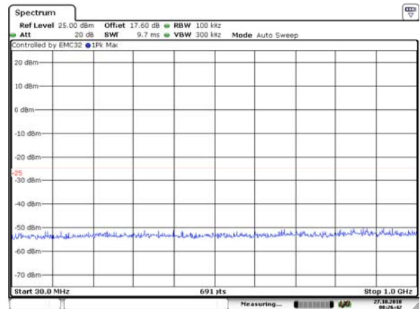
CA_41C 20MHz+20MHz CH- High 30MHz~1GHz
