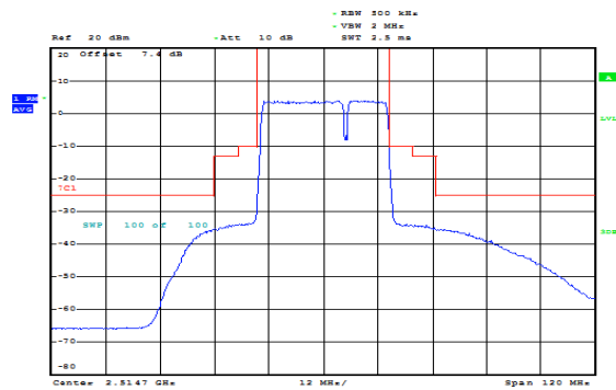
CA_7C 20MHz+10MHz QPSK RB=100#0+50#0 CH- Low
