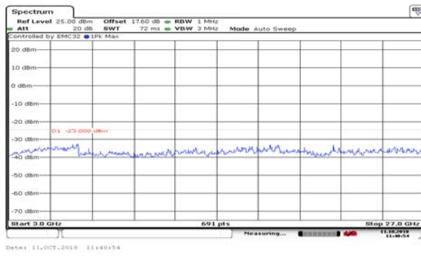
CA_7C 20MHz+10MHz CH- Middle 3GHz~27GHz
