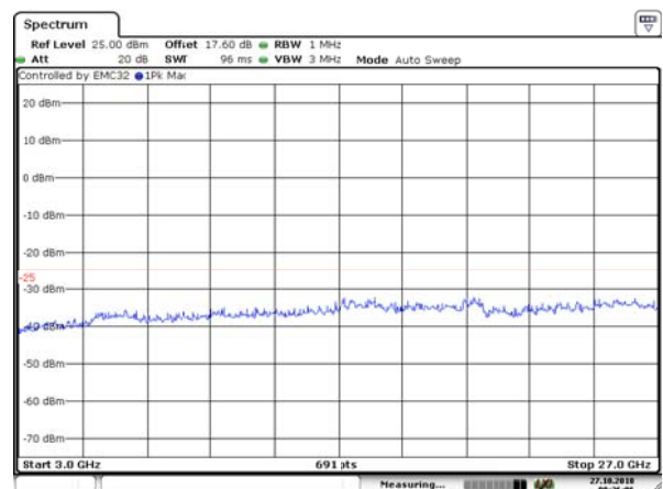
CA_41C 20MHz+20MHz CH- High 3GHz~27GHz
