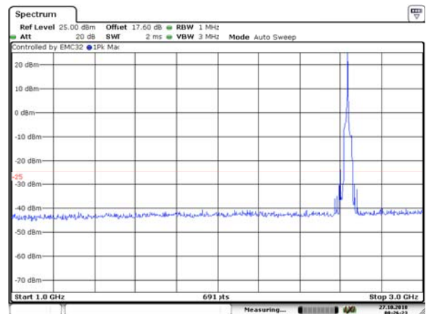
CA_41C 20MHz+20MHz CH- High 1GHz~3GHz
