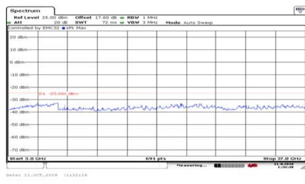
CA_7C 20MHz+10MHz CH-Low 3GHz~27GHz
