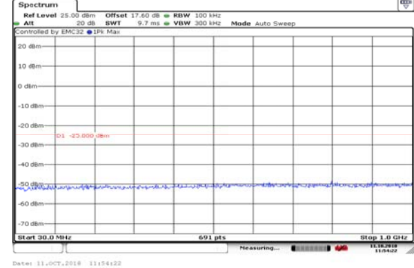
CA_7C 20MHz+20MHz CH-Low 30MHz~1GHz
