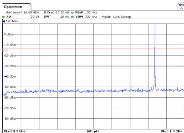
GSM 850 CH-Middle 9KHz ~ 1GHz
