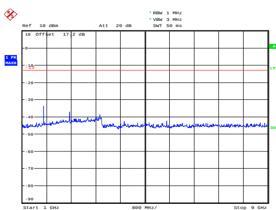
GSM 850 CH-High 1GHz ~ 9GHz
