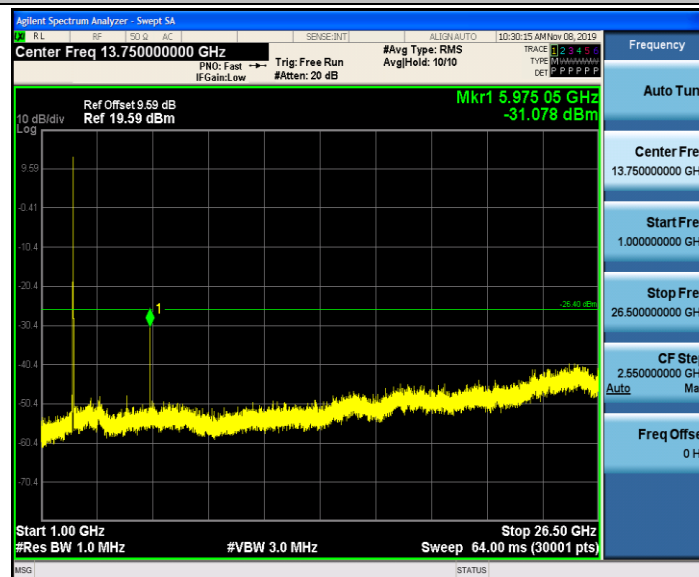
11N20MIMO_Ant1_2412_0~Reference
