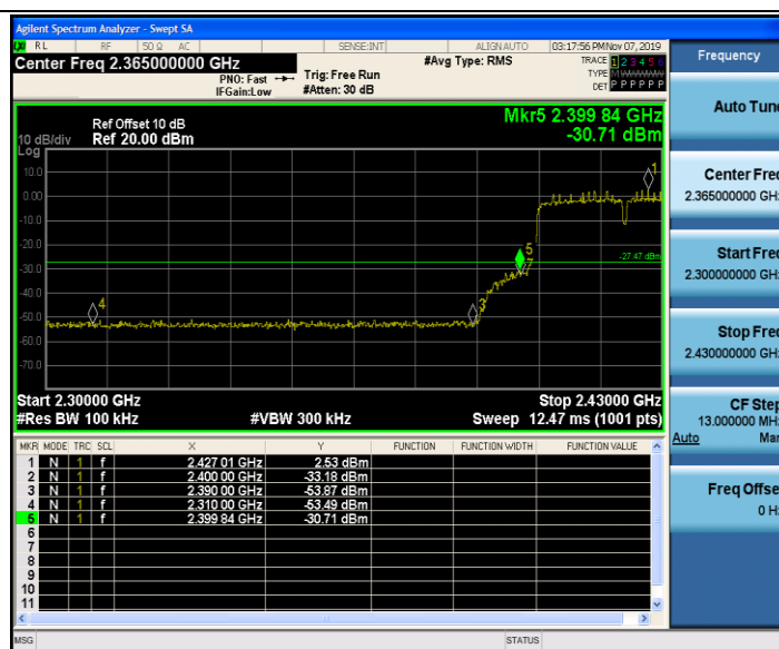
11N40SISO_Ant2_Low_2422
