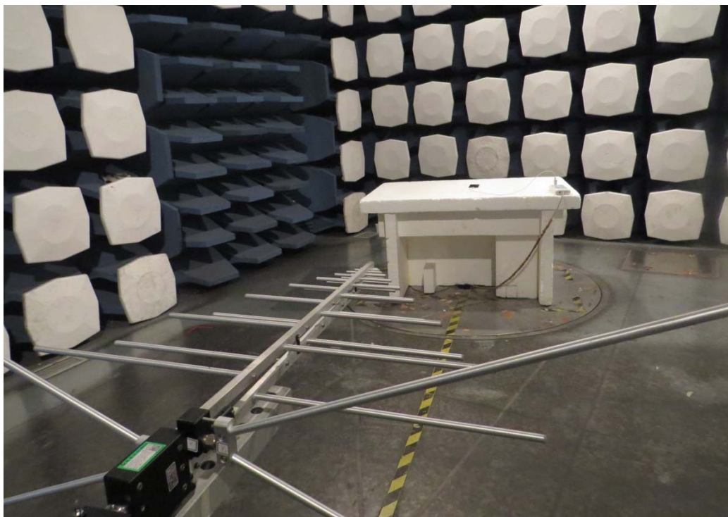
30MHz - 1GHz
