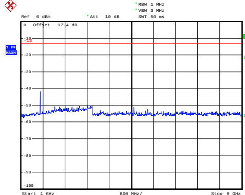
GSM 850 CH-High 1GHz ~ 9GHz
