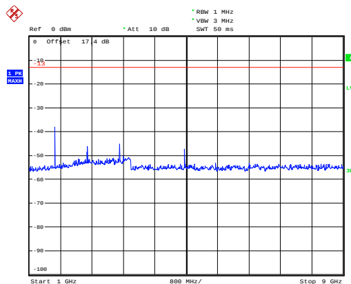
GSM 850 CH-Low 1GHz ~ 9GHz
