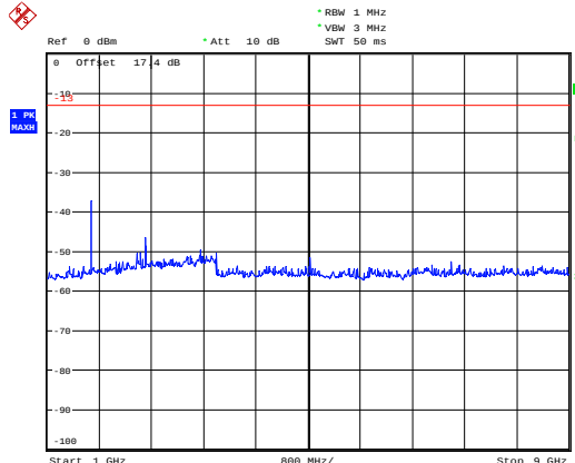
GSM 850 CH-Middle 1GHz ~ 9GHz
