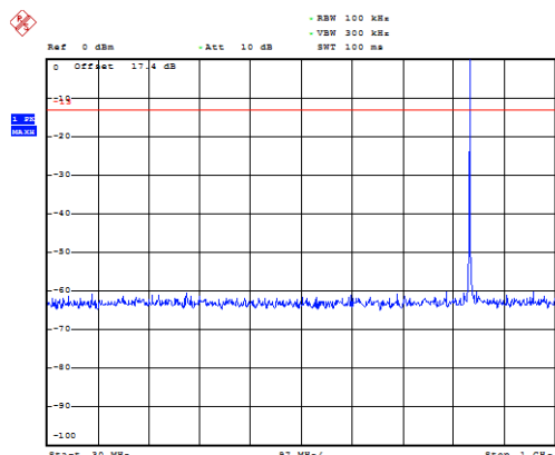
GSM 850 CH-Middle 30MHz ~ 1GHz
