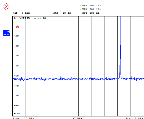
GSM 850 CH-Low 30MHz ~ 1GHz
