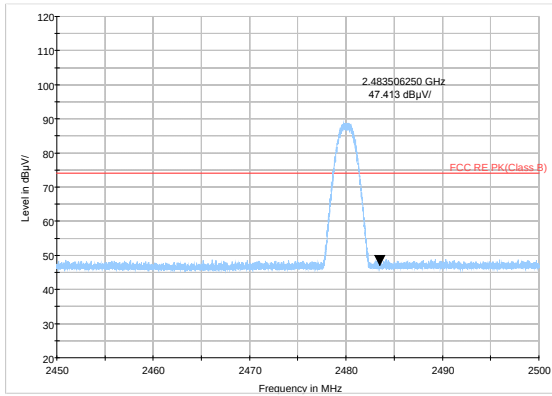
BLE V 5.0 Channel 39 Peak
