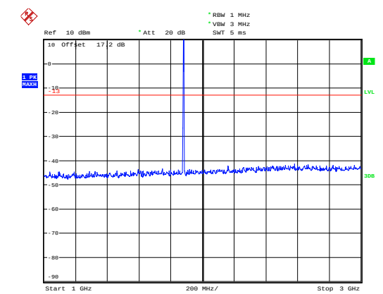
GSM 1900 CH-Middle 1GHz~3GHz
