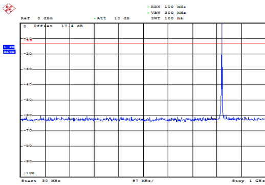
GSM 850 CH-Low 30MHz ~ 1GHz
