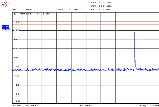
GSM 850 CH-Middle 30MHz ~ 1GHz
