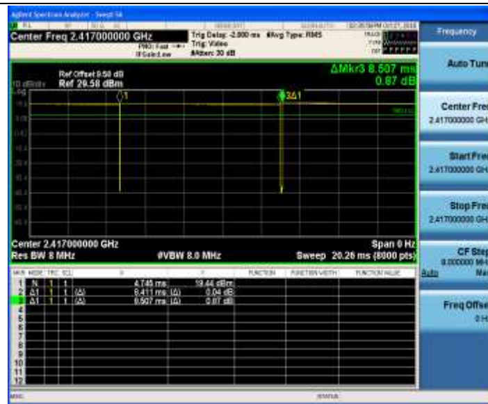
11B_Ant2_2417
