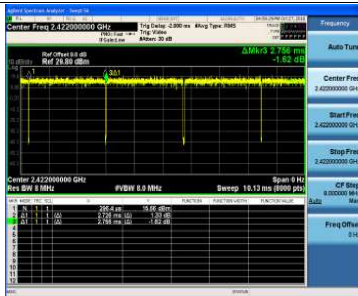
11G_Ant2_2422
