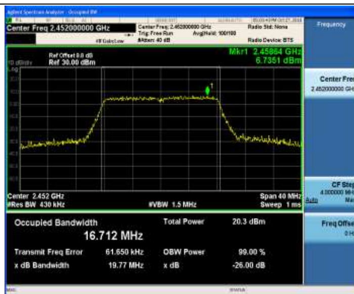
11G_Ant2_2452
