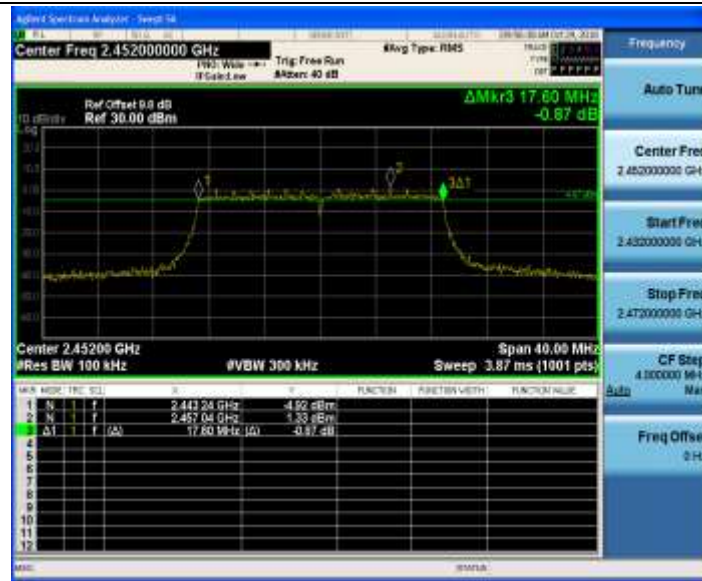
11N20MIMO_Ant2_2452
