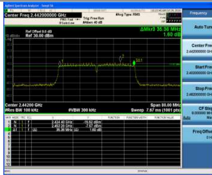
11N40MIMO_Ant2_2442
