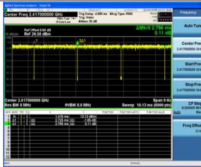
11G_Ant2_2417
