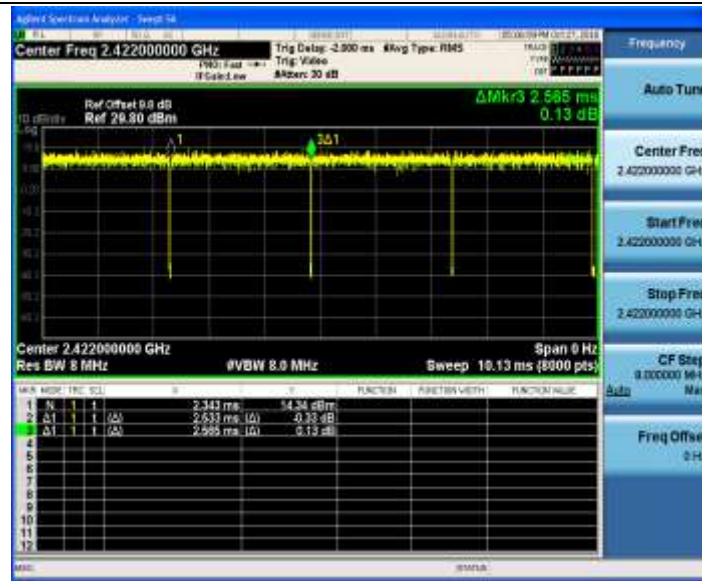
11N20SISO_Ant2_2422
