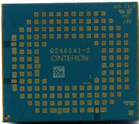
PVS8 Bottom Side
