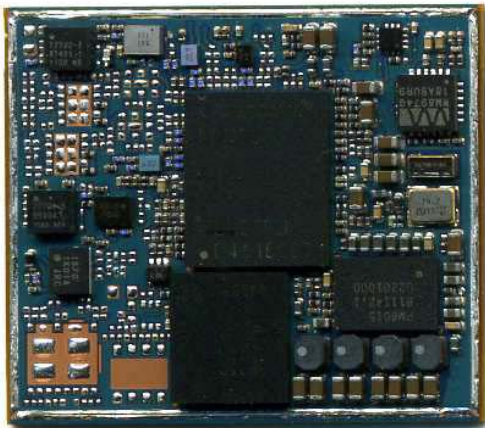
PVS8 Top side
