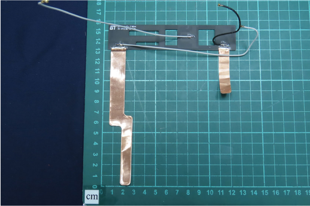
(26) EUT Photo_(Antenna)
