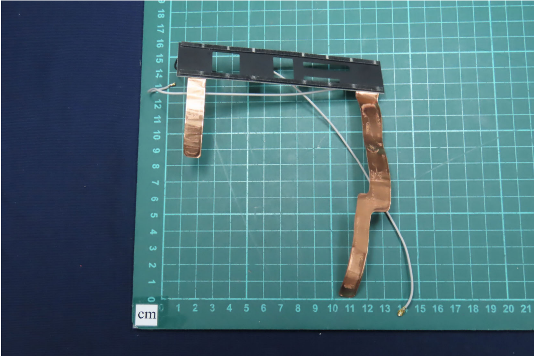
(27) EUT Photo_(Antenna)
