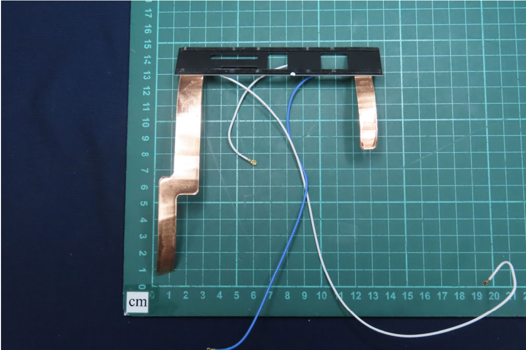
(25) EUT Photo_(Antenna)
