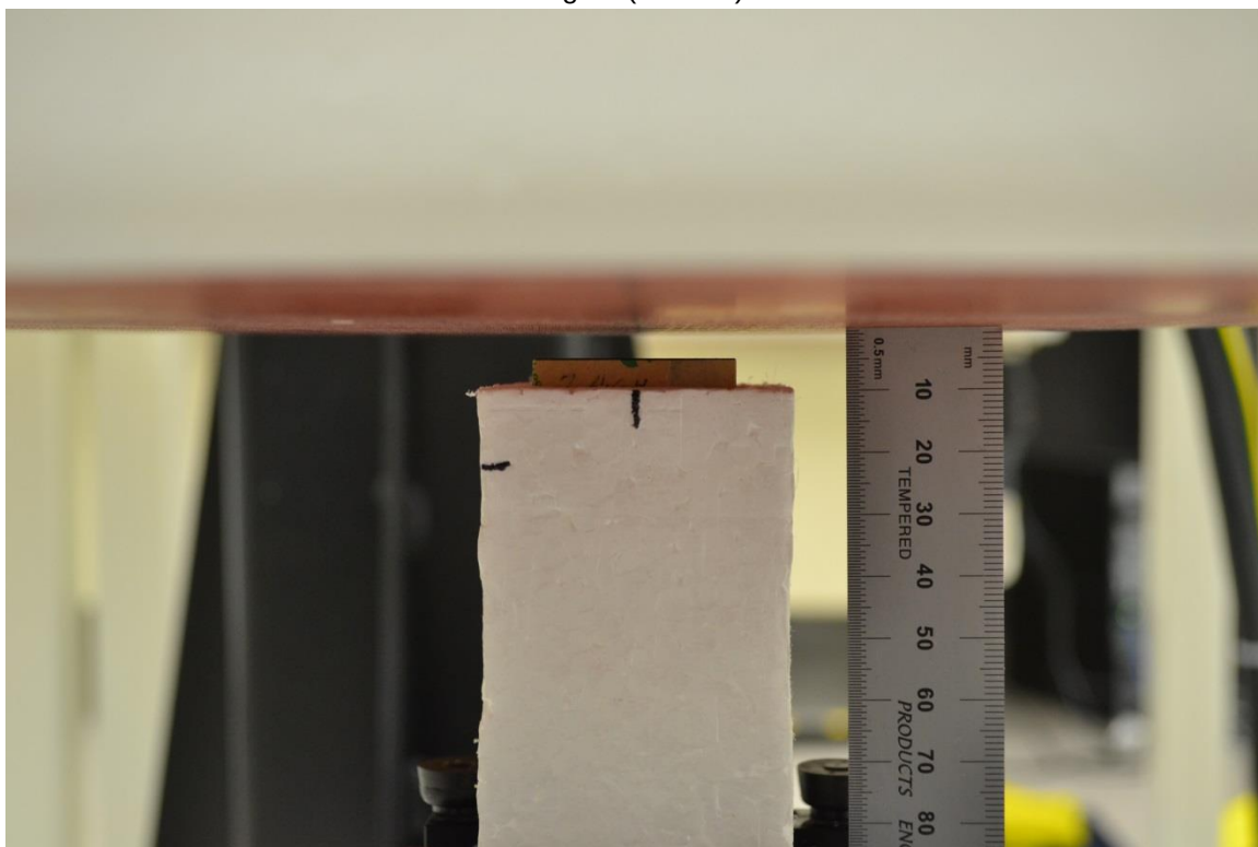
Edge 3 (5GHz)
