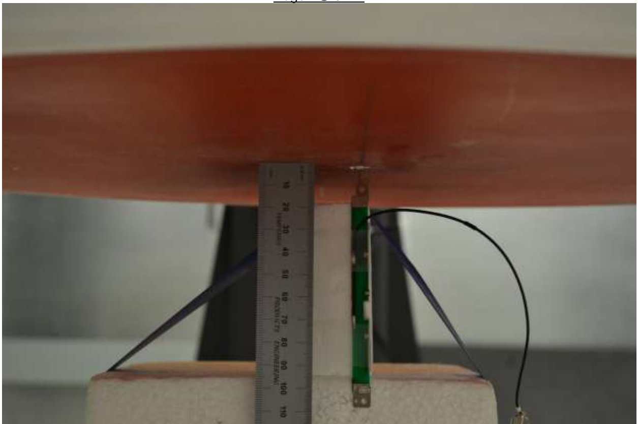
Edge 4 @ 5mm
