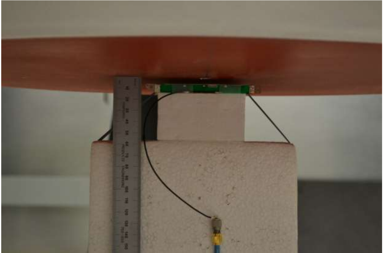
Edge 2 @ 5mm
