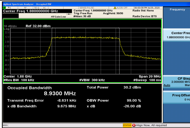
Band2-10MHz-QPSK-18900-50RB#0-8.9300
