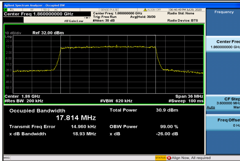
Band2-20MHz-QPSK-18700-100RB#0-17.814
