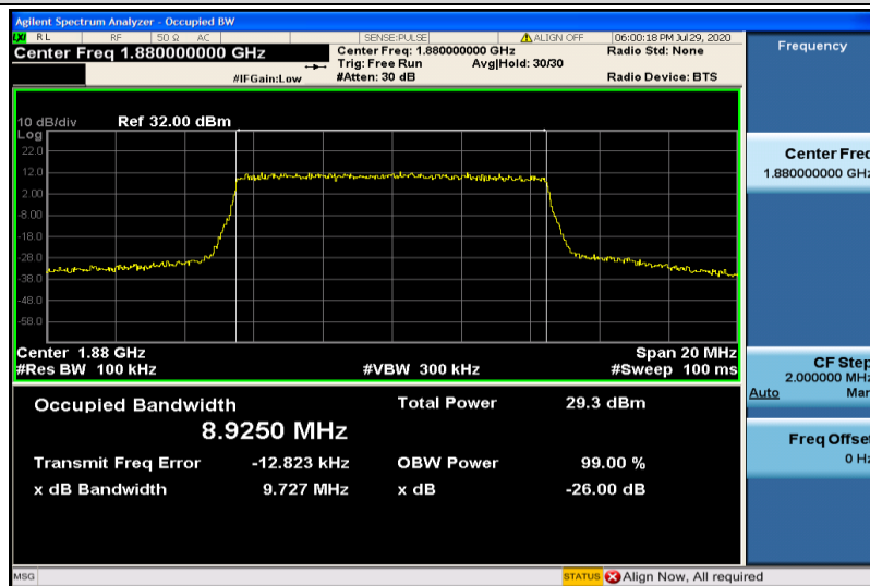
Band2-10MHz-16QAM-18900-50RB#0-8.9250
