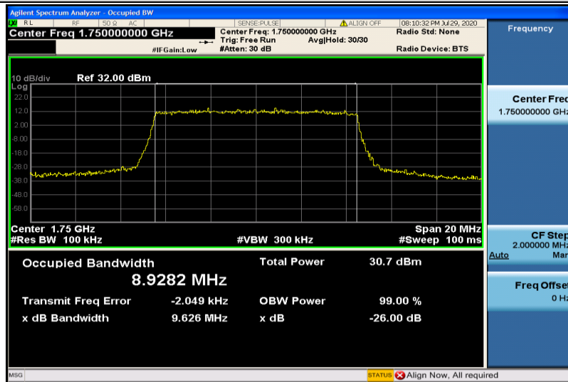
Band4-10MHz-QPSK-20350-50RB#0-8.9282
