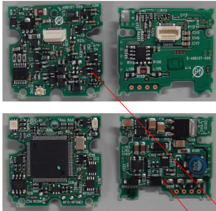
PCB_Main
