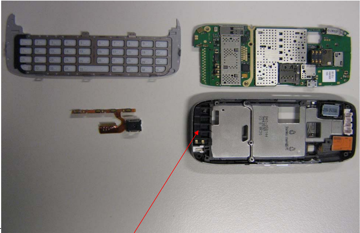
GSM/WCDMA Antenna
