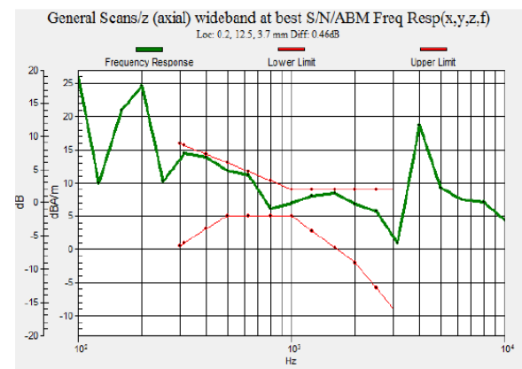
Fig. 7.12 WCDMA Band II Ch9538
