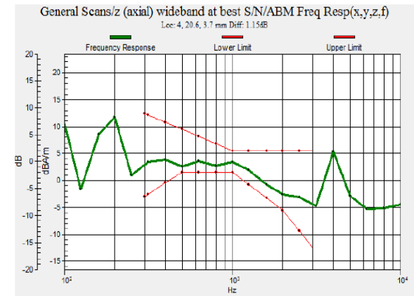
Fig. 7.10 WCDMA Band II Ch9262
