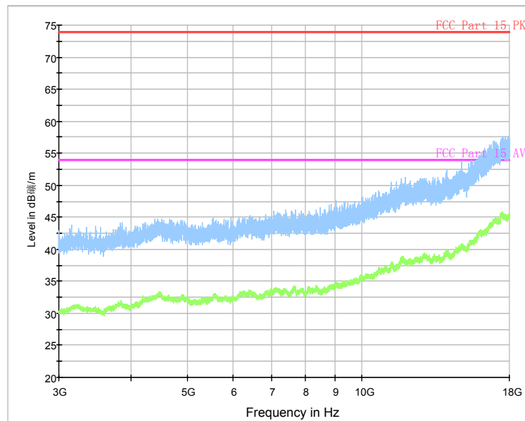
RE - 3GHz-18GHz
