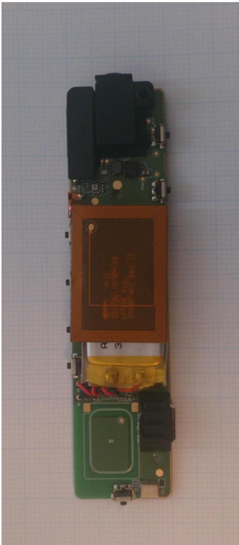
PCB rear side (NFC-antenna)
