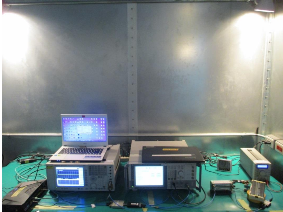
EUT
