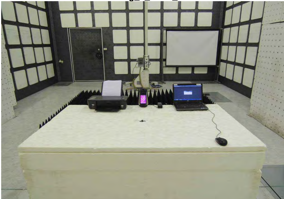
Config_1_Read_-
