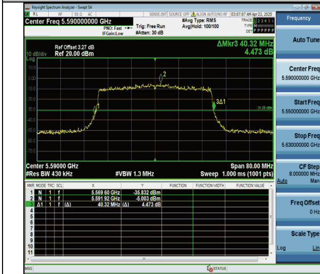
11ax40MIMO-Ant6-5590
