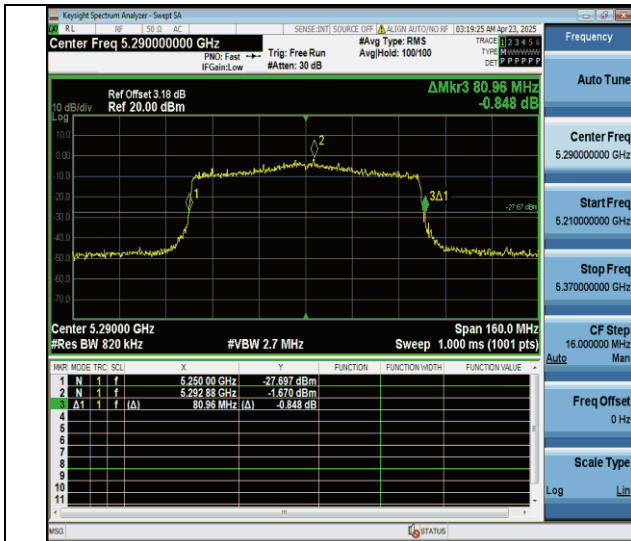
11ax80MIMO-Ant6-5290
