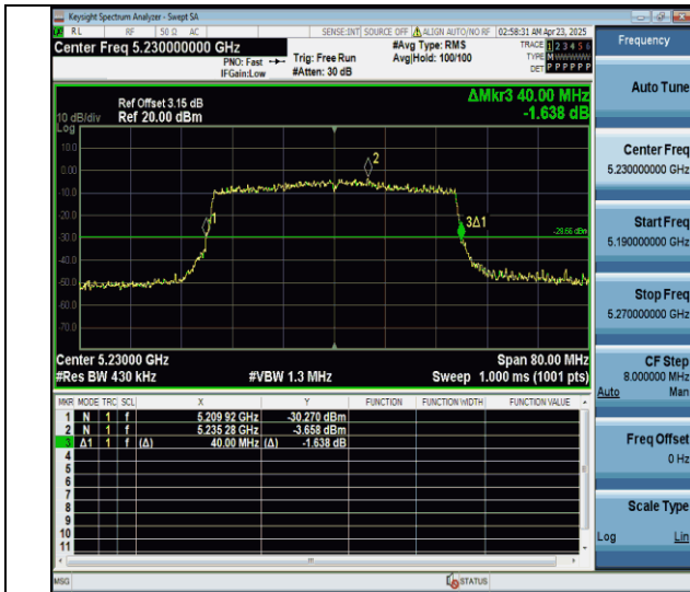
11ax40MIMO-Ant6-5230
