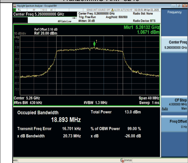
11ax20MIMO-Ant7-5260
