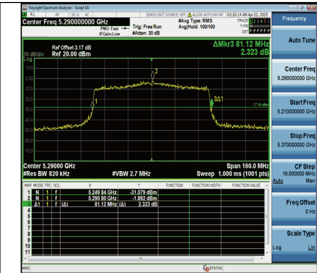
11ax80MIMO-Ant7-5290
