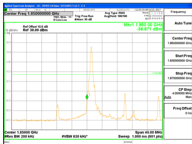
LTE B25 20MHz QPSK Low Channel 1RB
