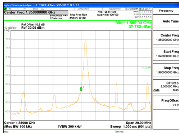
LTE B25 10MHz QPSK Low Channel 1RB
