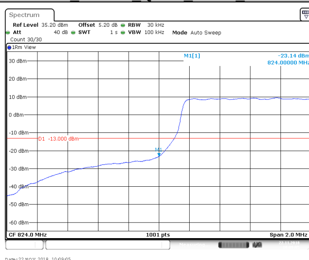
Band5 1.4MHz QPSK 20643 1RB#5
