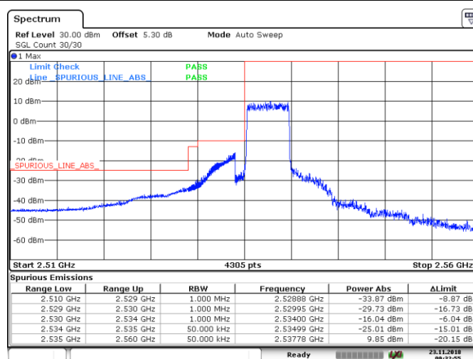
Band41_5MHz_QPSK_40065_25RB#0
