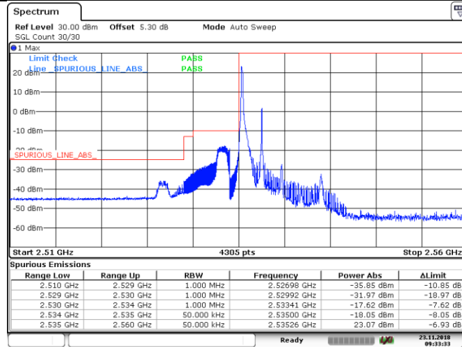
Band41_5MHz_QPSK_40065_1RB#0
