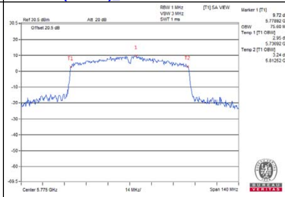
802.11ac (80MHz)_Chain 1 / CH 155
