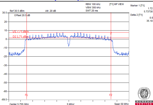
802.11ac (40MHz)_Chain 1 / CH 151
