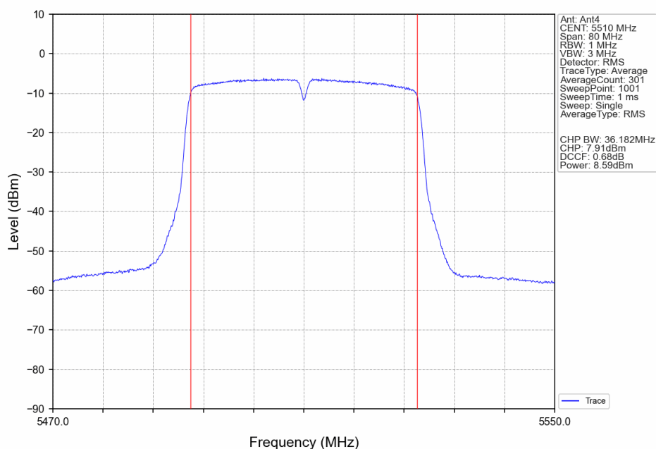
802.11n(HT40)_LCH_5510MHz_Ant4_NTNV
