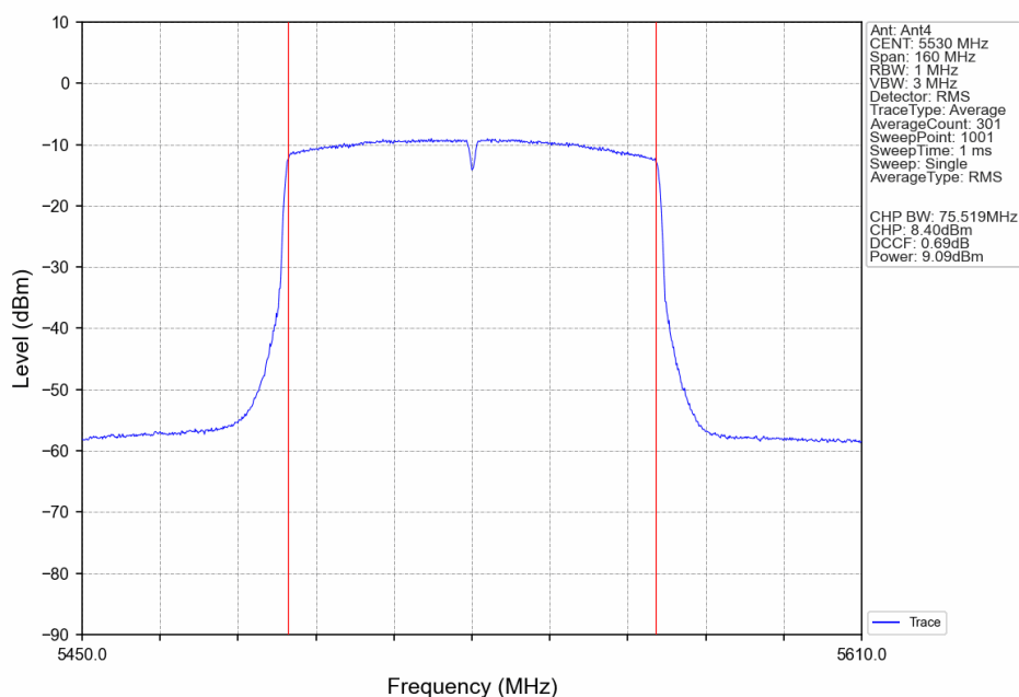
802.11ac(VHT80)_LCH_5530MHz_Ant4_NTNV
