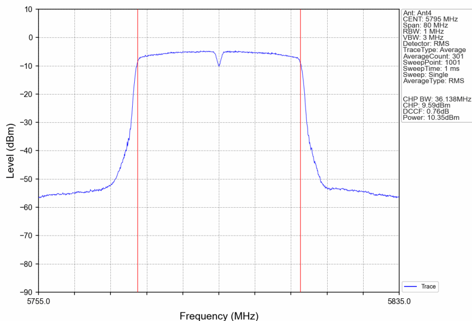
802.11n(HT40)_HCH_5795MHz_Ant4_NTNV
