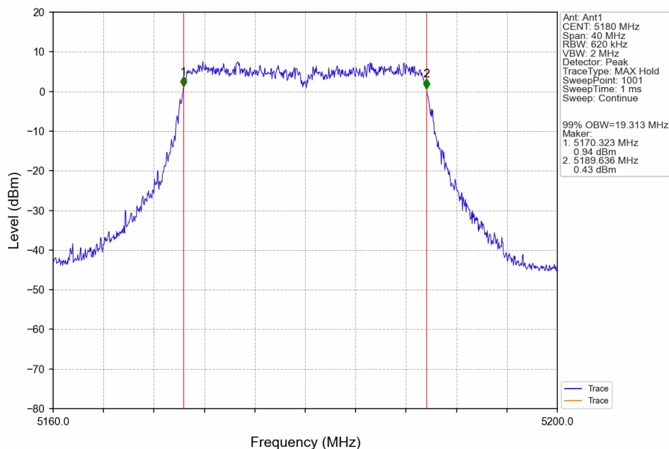
802.11ax(HEW20)_LCH_5180MHz_RU242_Left_Ant1_NTNV
