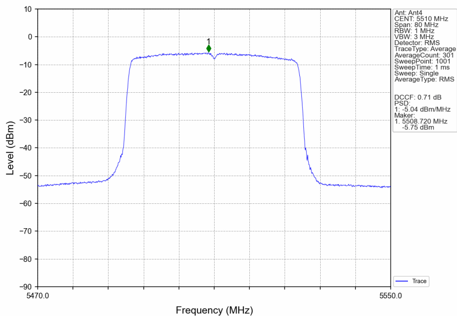
802.11ax(HEW40)_LCH_5510MHz_RU26_Left_Ant4_NTNV
