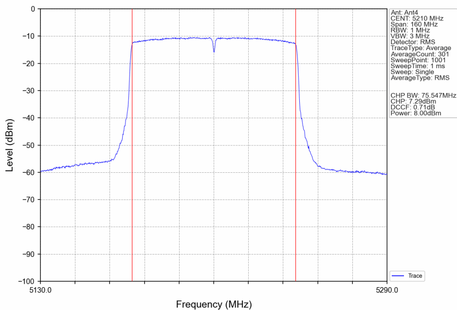
802.11ac(VHT80)_MCH_5210MHz_Ant4_NTNV
