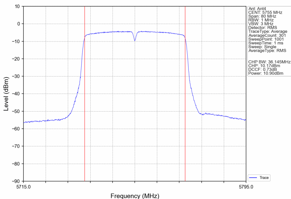
802.11n(HT40)_LCH_5755MHz_Ant4_NTNV
