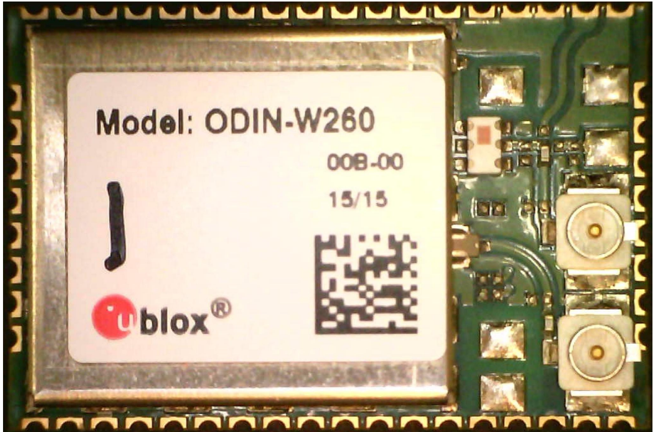
151496_07.jpg: EUT – Top View (Odin-W260)
