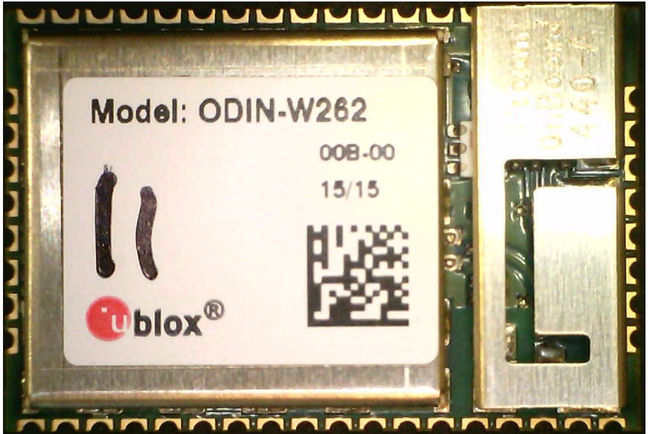
151496_08.jpg: EUT – Top View (Odin-W262)
