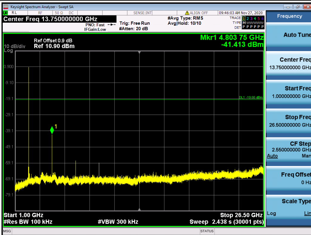
2DH5 Ant1 2402 1000~26500
