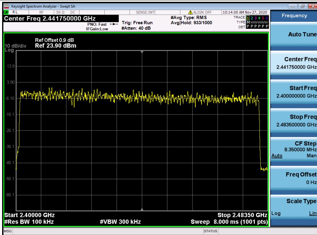
3DH5_Ant1_Hop
