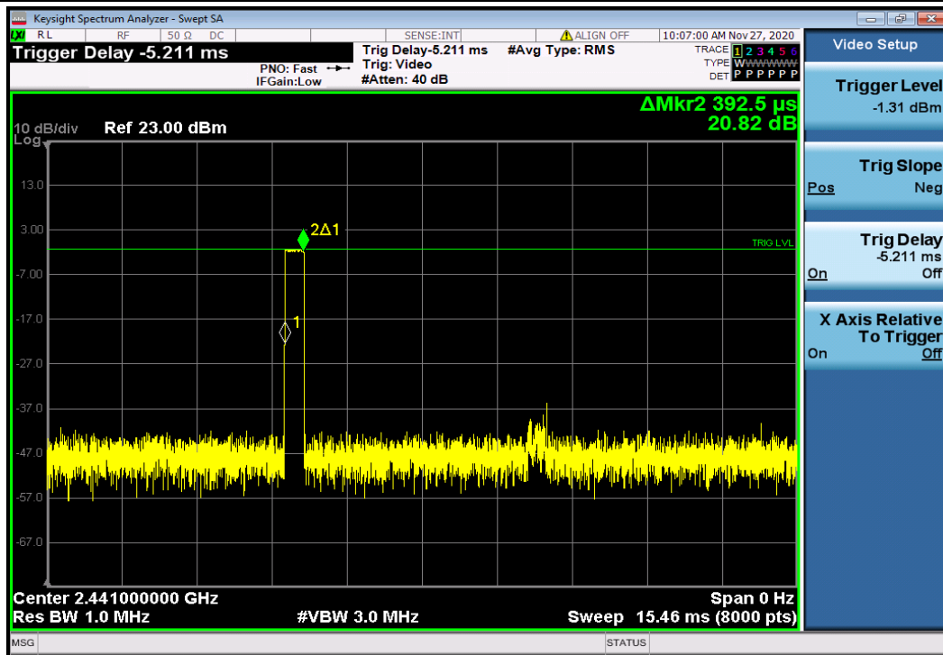
DH1_Ant1_Hop
