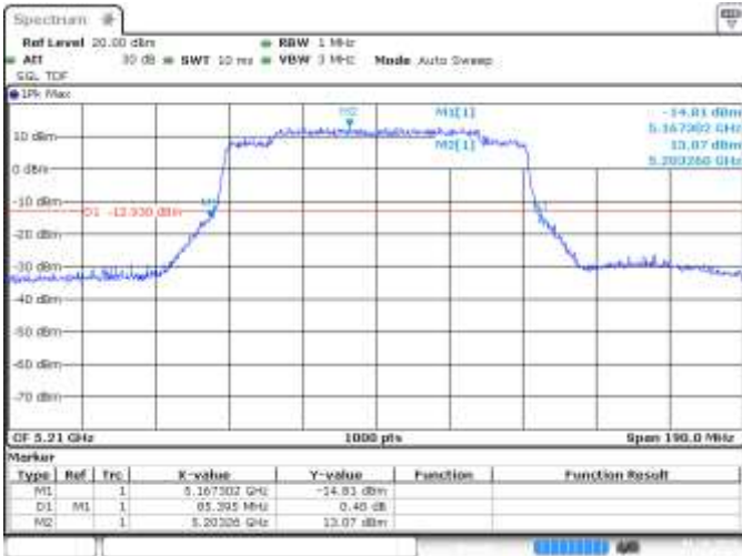
SISO B, CH42, 802.11ax80, HE0, 99% BW
