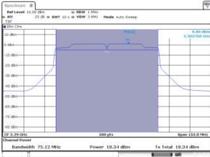
SISO A, 802.11ac80, CH58, VHT0
