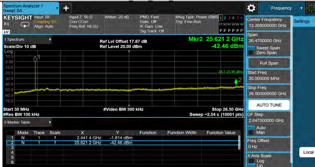
DH5 Ant1 2441 30~26500
