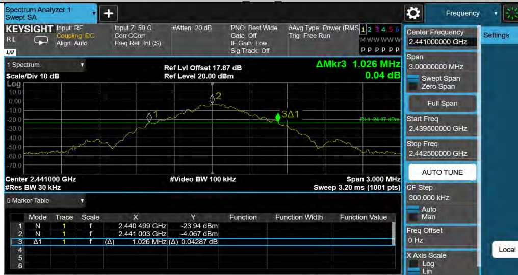
DH5 Ant1 2441
