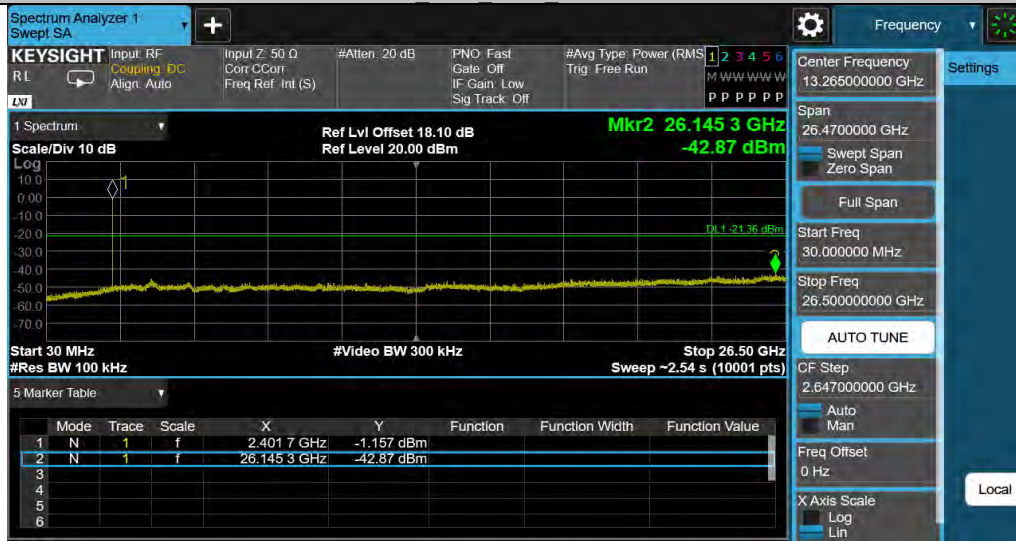
DH5 Ant1 2402 30~26500
