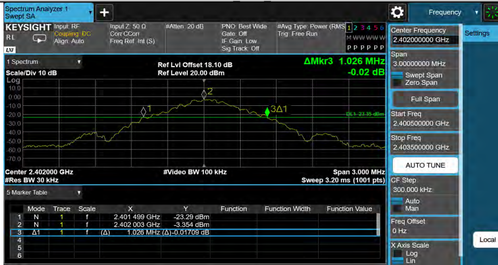
DH5 Ant1 2402
