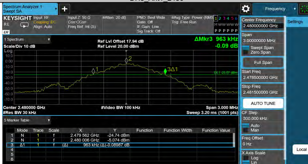
DH5 Ant1 2480
