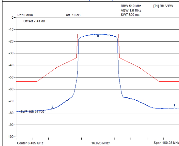
802.11ax (HE40) / Chain 0 : CH 91
