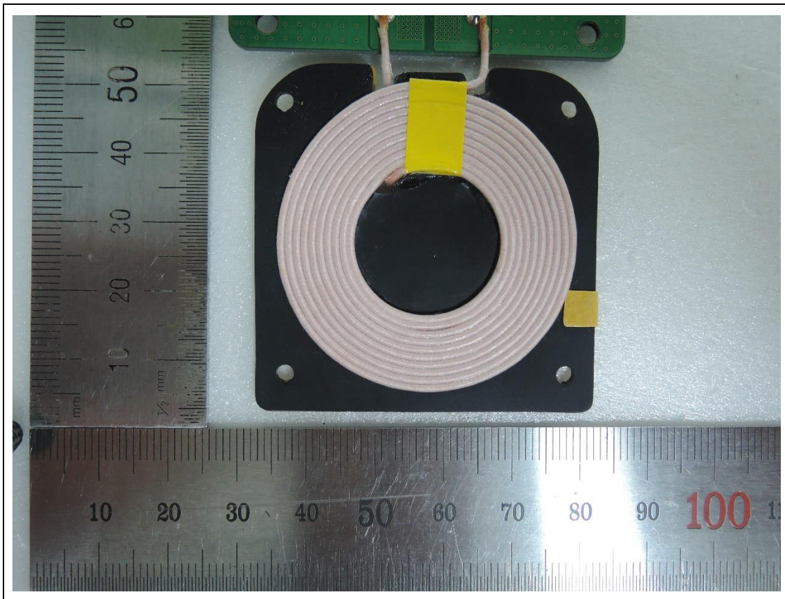
&lt;Antenna&gt;
