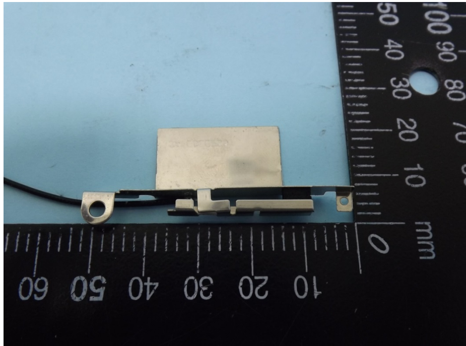
PIFA Antenna
