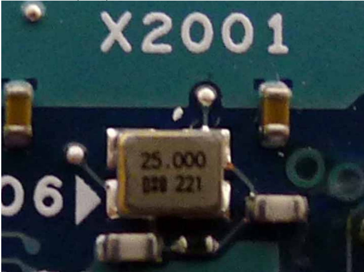
EUT-29. 25MHz(X2001)
