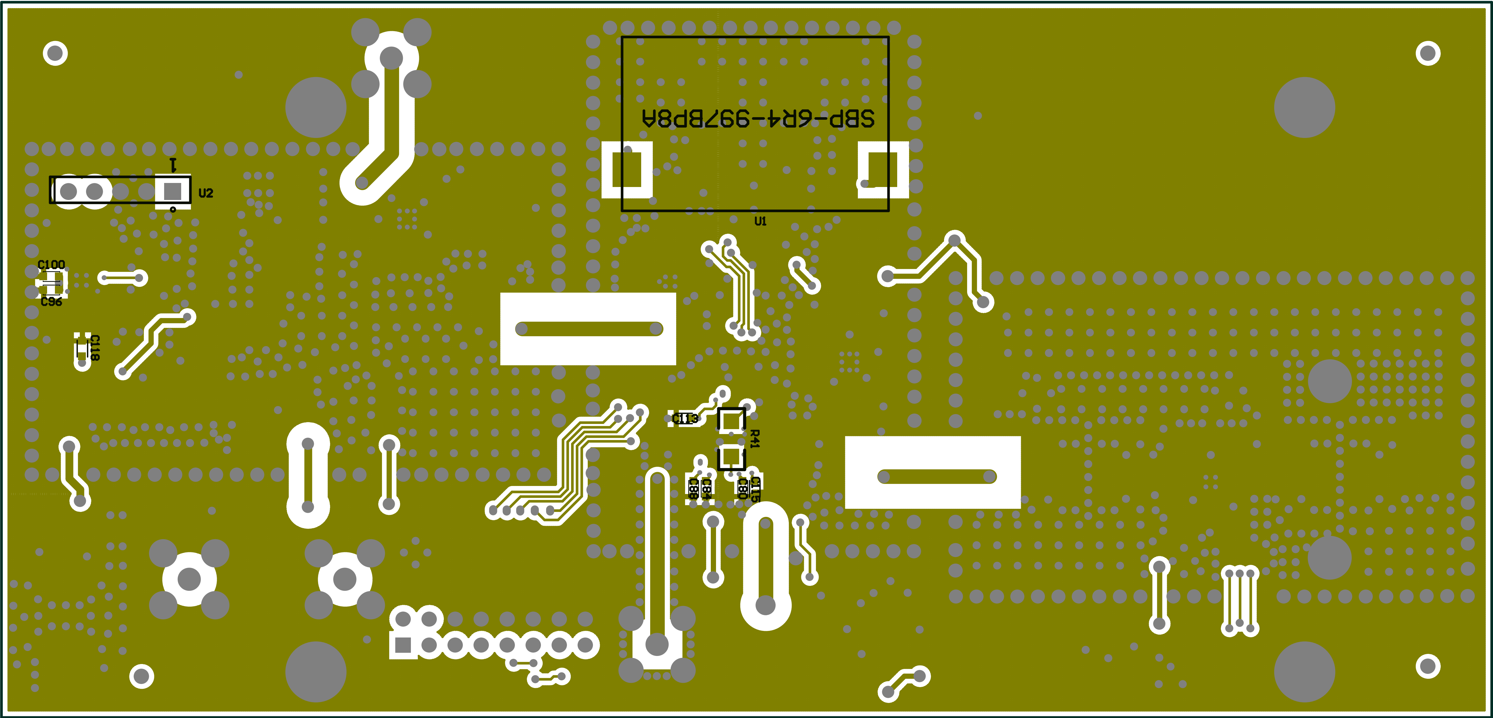
Bottom Layer Bottom Overlay
