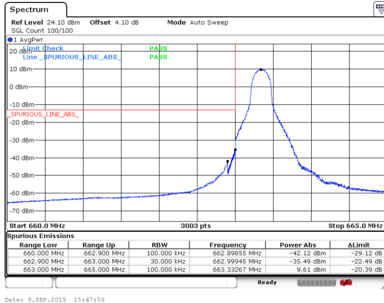
Band71-5MHz-QPSK-133147-25RB#0
