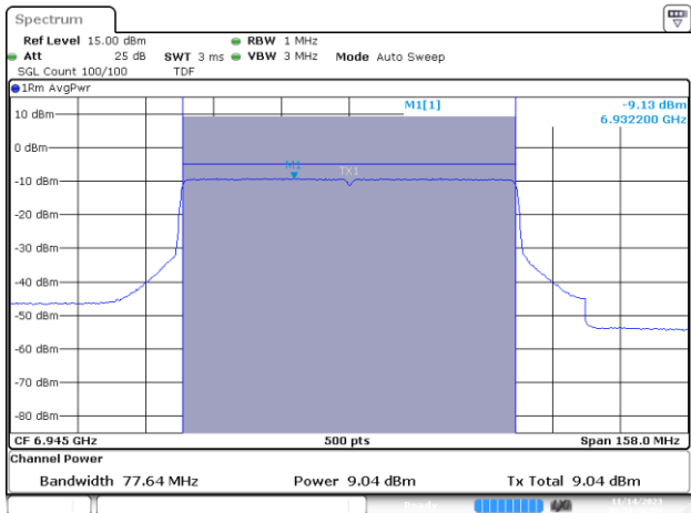
MIMO B-802.11ax/be-80MHz-Ch199-6945MHz-MCS0
