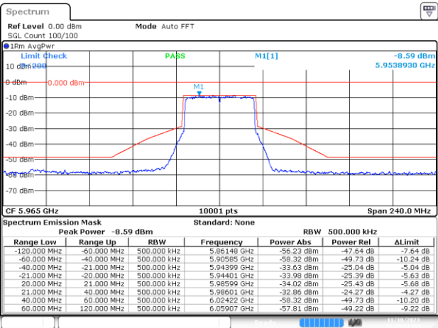
SISO A-802.11ax/be-40MHz-Ch3-5965MHz-MCS0
