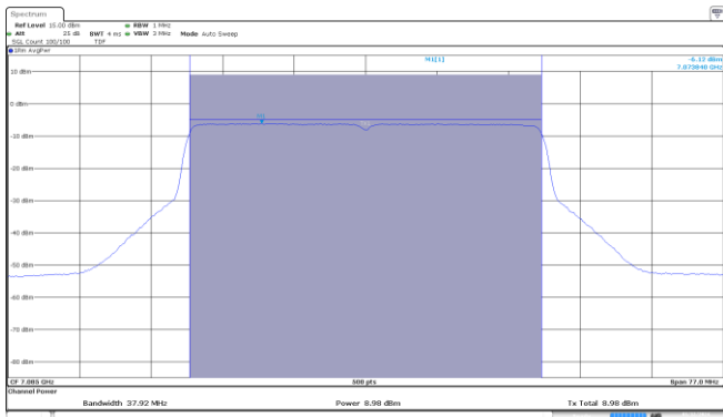
SISO A-802.11ax/be-40MHz-Ch227-7085MHz-MCS0
