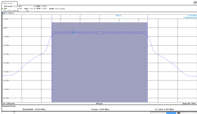
SISO A-802.11ax/be-20MHz-Ch229-7095MHz-MCS0
