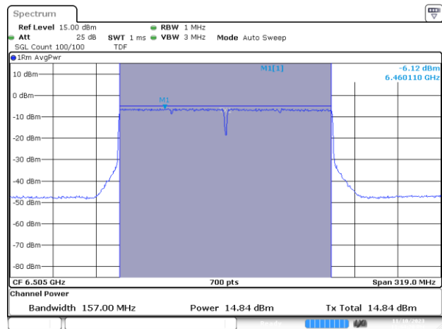
SISO A-802.11ax/be-160MHz-Ch111-6505MHz-MCS0
