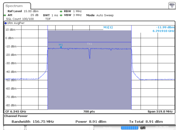
SISO B-802.11ax/be-160MHz-Ch79-6345MHz-MCS0
