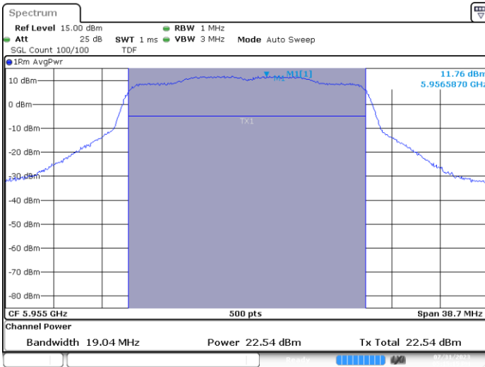
SISO A-802.11ax/be-20MHz-Ch1-5955MHz-MCS0
