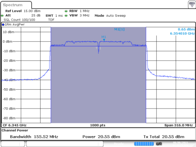
MIMO A-802.11ax/be-160MHz-Ch79-6345MHz-MCS0
