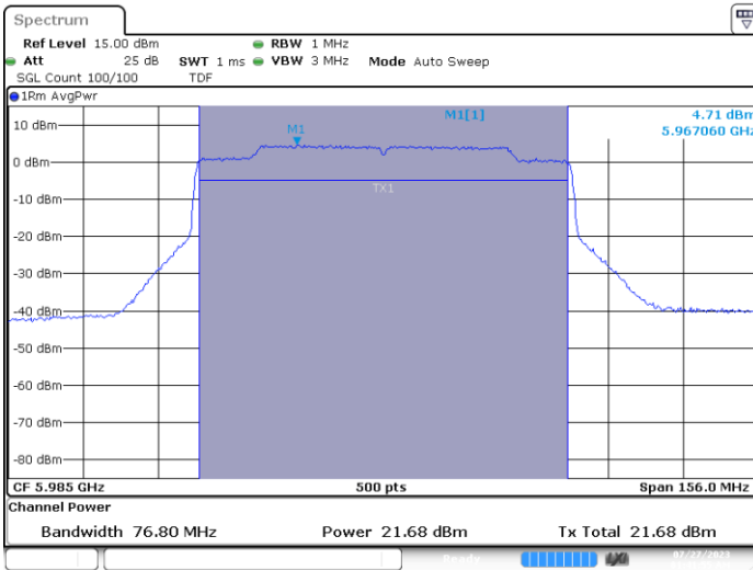
MIMO A-802.11ax/be-80MHz-Ch7-5985MHz-MCS0
