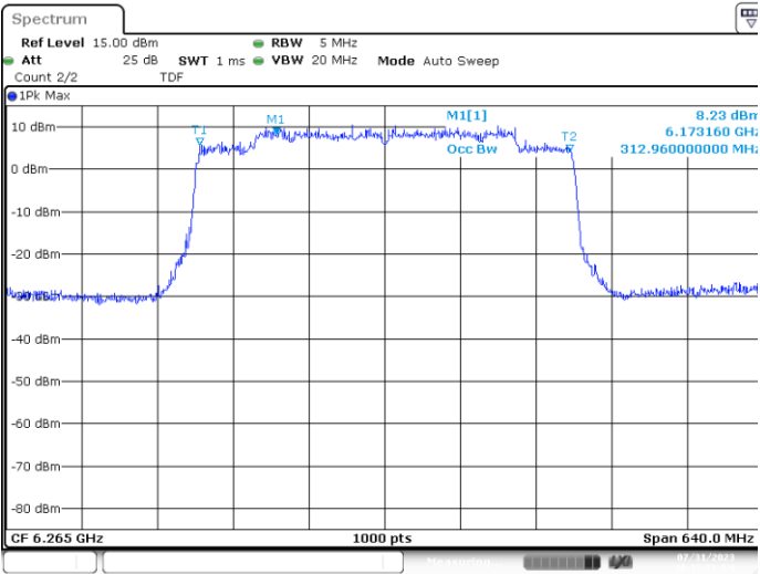
UNII6 MIMO B 802.11be320 ch63 6265MHz 99%
