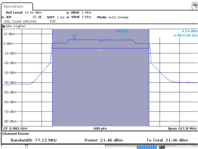
MIMO B-802.11ax/be-80MHz-Ch7-5985MHz-MCS0
