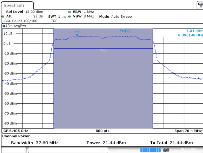
MIMO B-802.11ax/be-40MHz-Ch91-6405MHz-MCS0
