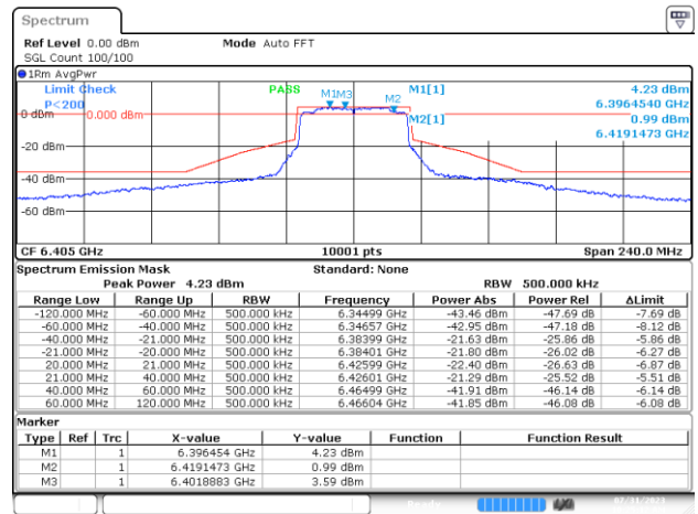
MIMO B-802.11ax/be-40MHz-Ch91-6405MHz-MCS0
