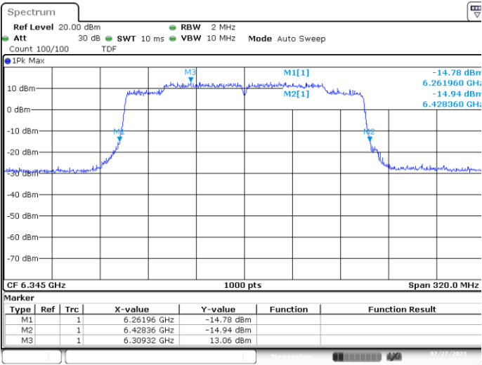
UNII5 MIMO A 802.11ax/be160 ch79 6345MHz 26dB
