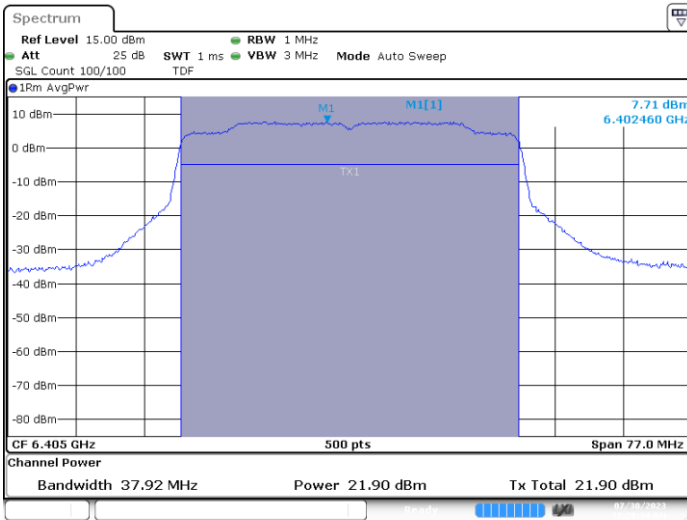
MIMO A-802.11ax/be-40MHz-Ch91-6405MHz-MCS0
