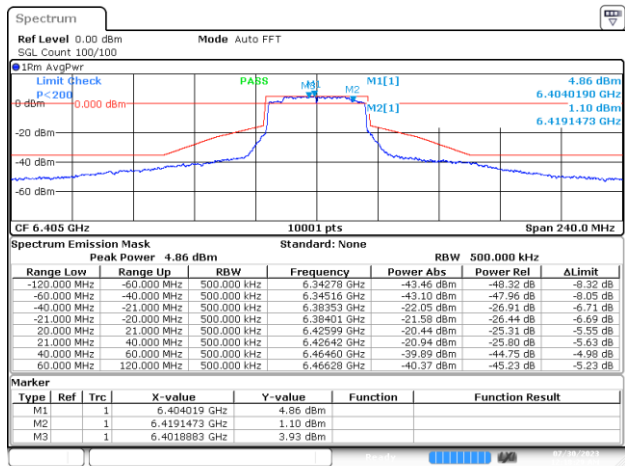
MIMO A-802.11ax/be-40MHz-Ch91-6405MHz-MCS0
