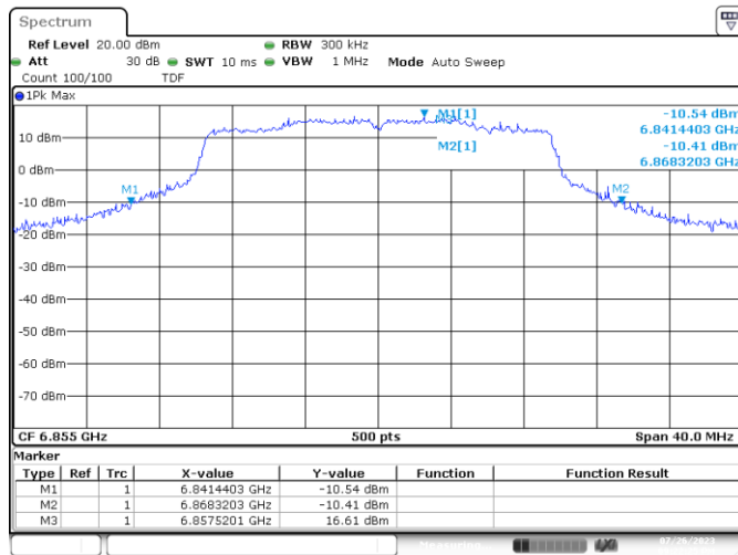
UNII7 SISO 802.11ax/be20 ch181 6855MHz 26dB
