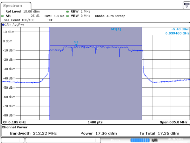
MIMO B-802.11be-320MHz-Ch31-6105MHz-MCS0
