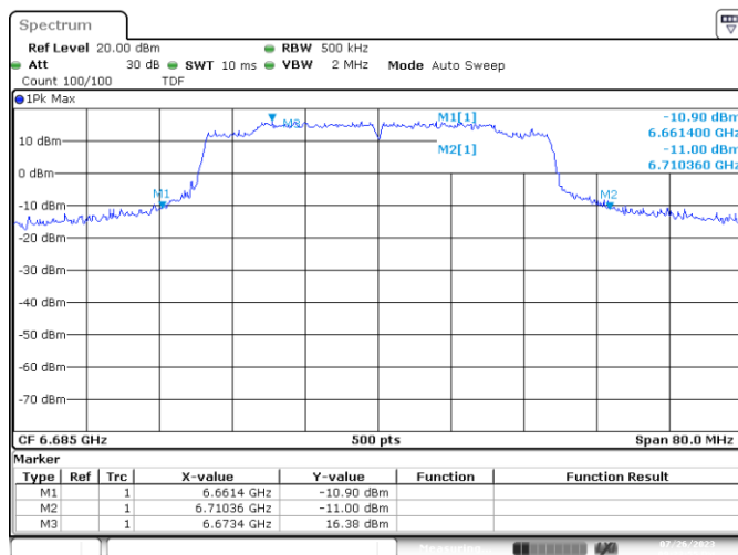
UNII7 SISO A 802.11ax/be40 ch147 6685MHz 26dB
