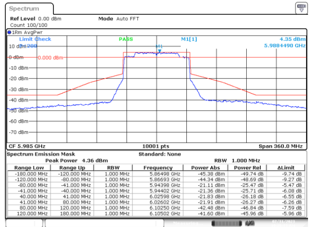
MIMO B-802.11ax/be-80MHz-Ch7-5985MHz-MCS0
