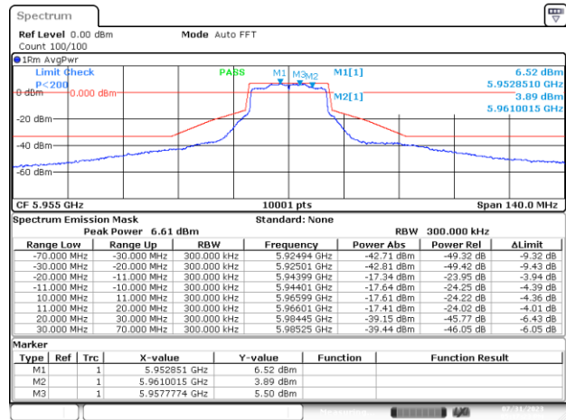
SISO A-802.11ax/be-20MHz-Ch1-5955MHz-MCS0
