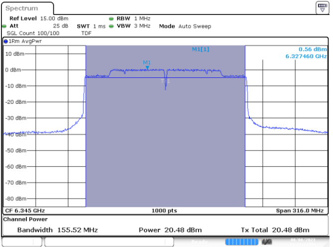
MIMO B-802.11ax/be-160MHz-Ch79-6375MHz-MCS0
