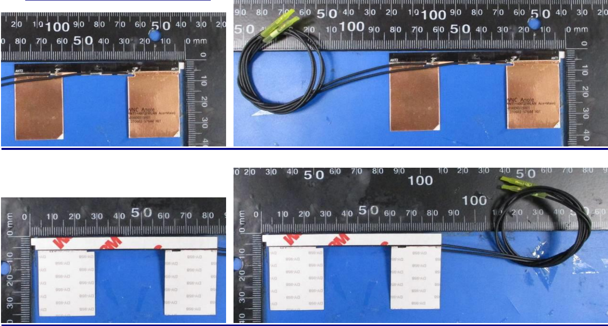
Tx1 (AUX) Antenna Photo:
